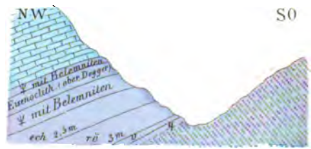
Fig. 10. Querprofil am Contact an der Orftlah ( Mettenberg )
